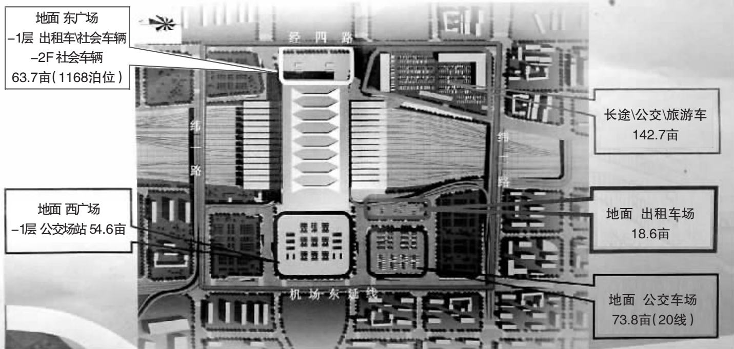
沙河堡铁路新客站站区布局
